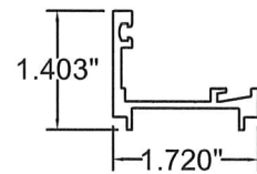
25 Gutter 6063-T5
