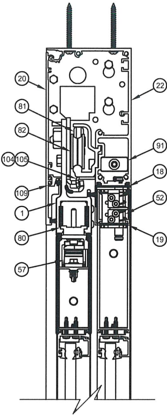
Section A-A
