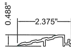
5 Leadup 6063-T5
