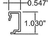
24 9/16" Snap 6063-T5
