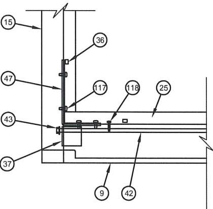
Sidelite Bottom Jamb Corner
