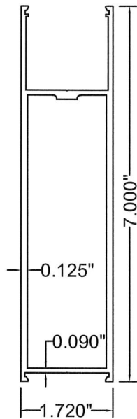
11 H7 6063-T5
