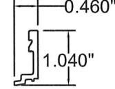
23 1" Snap 6063-T6
