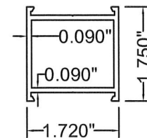
8 H2 6063-T5
