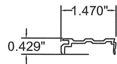
6 Filler 6063-T5
